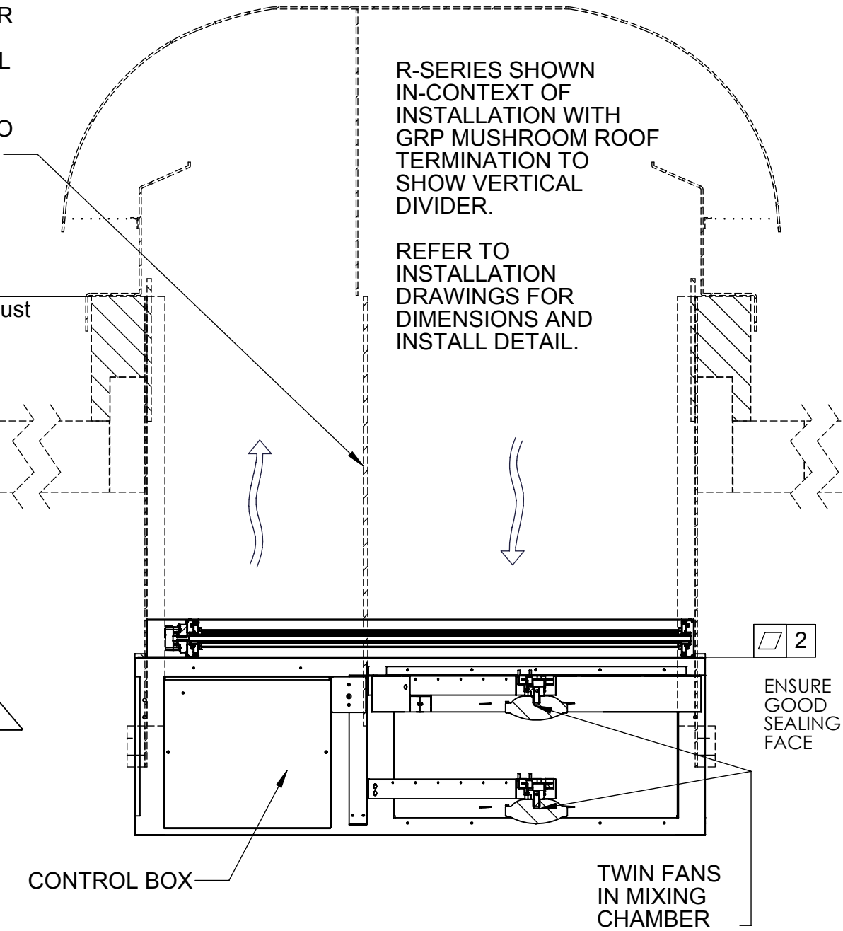
SECTION A-A
